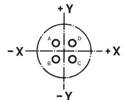
8 – 4 4 Kontakte Größe 20
