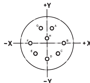
12 – 8 8 Kontakte Größe 20
