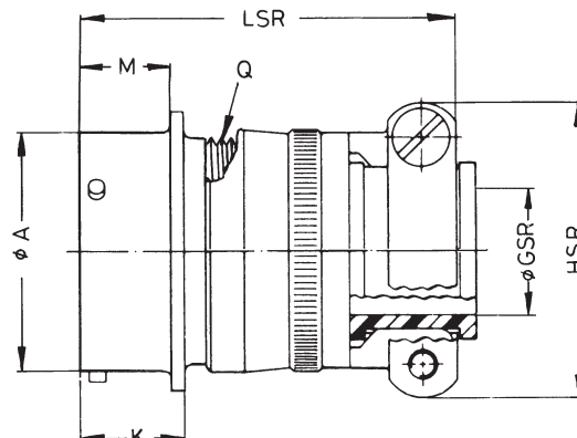
PT 01 A ... SR PT 01 E ... SR (MS 3110 F) PT 01 P ... SR
