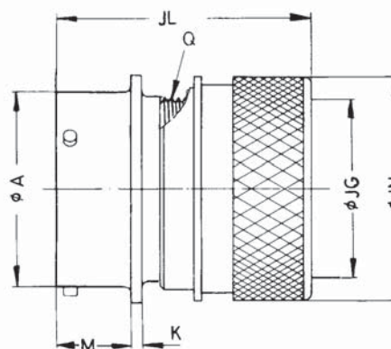
PT 00 SE ... J
