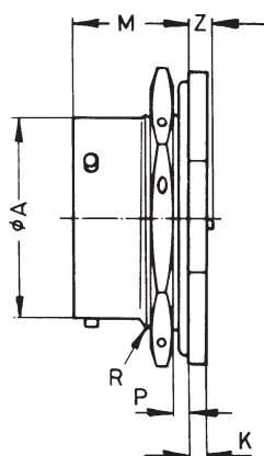
PT 07 H (VG 95328 F / MS 3114 H)
