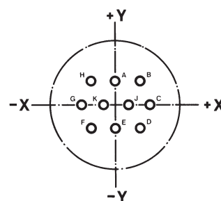
12 – 10 10 Kontakte Größe 20
