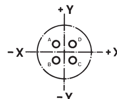
8 – 4 4 Kontakte Größe 20
