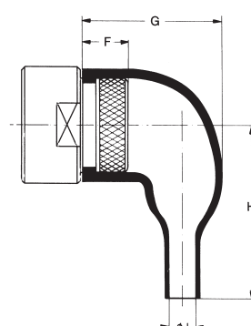
Endgehäuse SE ... F mit Formteil 222
