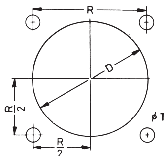
Montagebohrung
