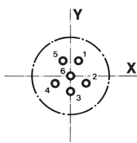
8-35 6 Kontakte Größe 22D
