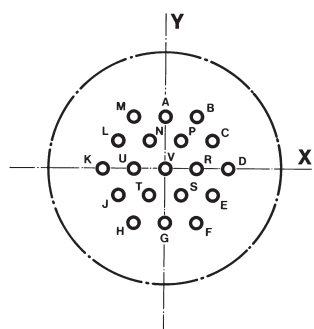
14-19 19 Kontakte Größe 20
