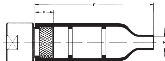
Gehäuseabschluss F mit Formteil 202
