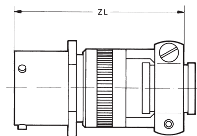
Kabelverbindungsstecker mit Zugentlastungsschelle (s. S. 27)
