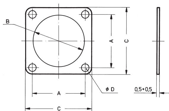
Flanschdichtung 10-101949 (VG 95328 T 0 7 A)
