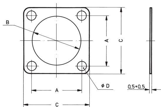
Flanschdichtung mit Schirmgeflecht 10-40450 (VG 95328 T 0 7 B)
