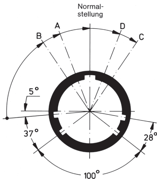
Vorderansicht einer Steckdose
