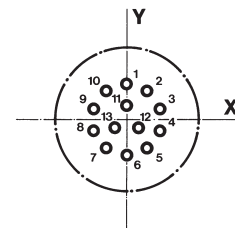
10-35 13 Kontakte Größe 22D
