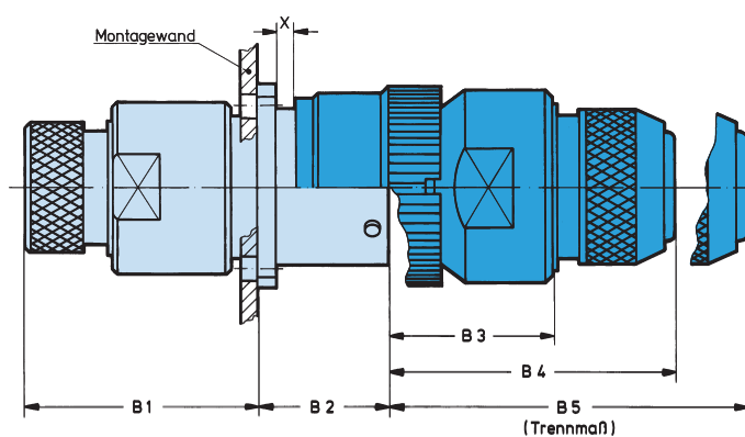
SJT 00 RT mit Gehäuseabschluss F
