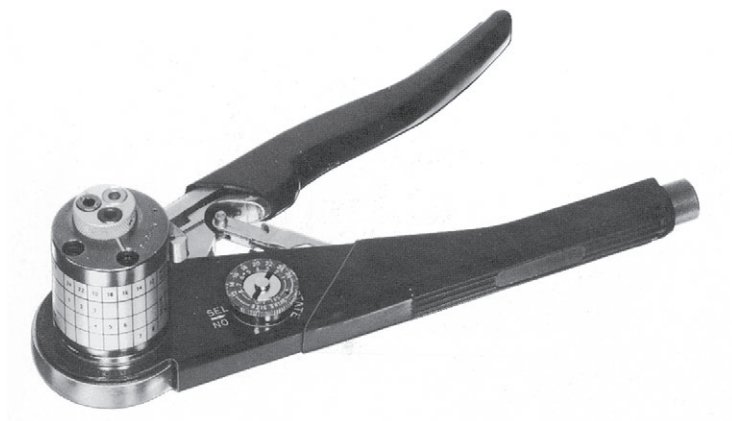
Crimp-Zange M 22520/1-01 (8-Kerb-Crimpverbindung)
