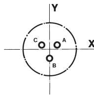
8-98 3 Kontakte Größe 20
