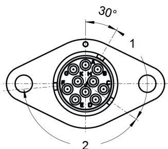
Receptacle
