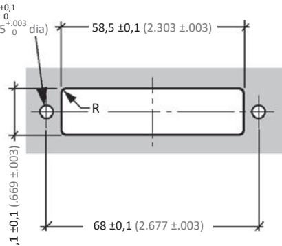
Montage par l'arrière (pour PCB) Rear mounting (for PCB)
