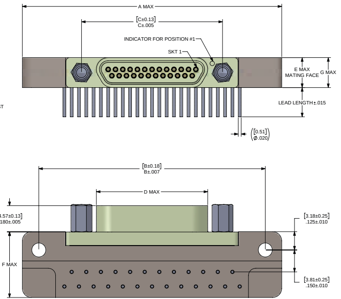
RECEPTACLE
