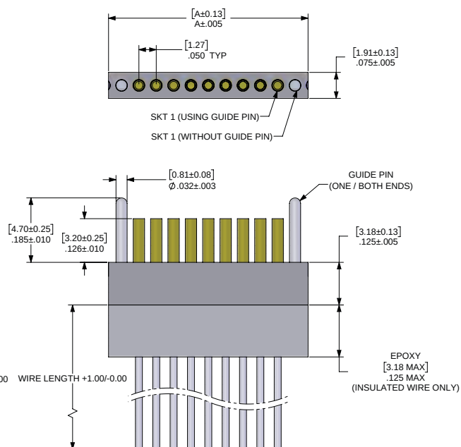
RECEPTACLE
