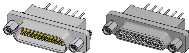
RECEPTACLE
