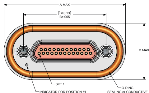
RECEPTACLE
