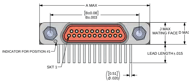
RECEPTACLE
