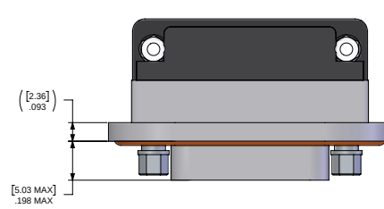
RECEPTACLE
