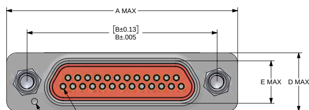
RECEPTACLE
