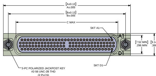
RECEPTACLE
