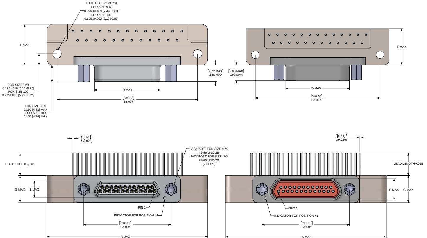
RECEPTACLE
