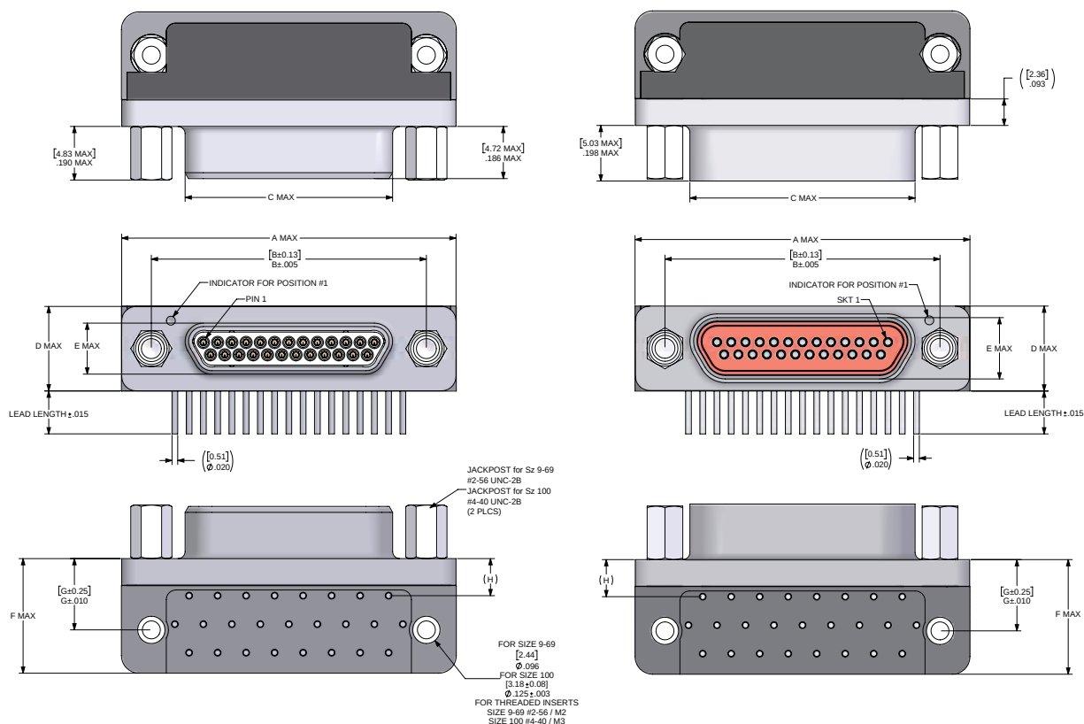
RECEPTACLE
