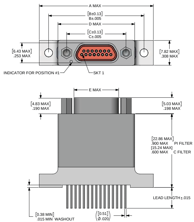
RECEPTACLE
